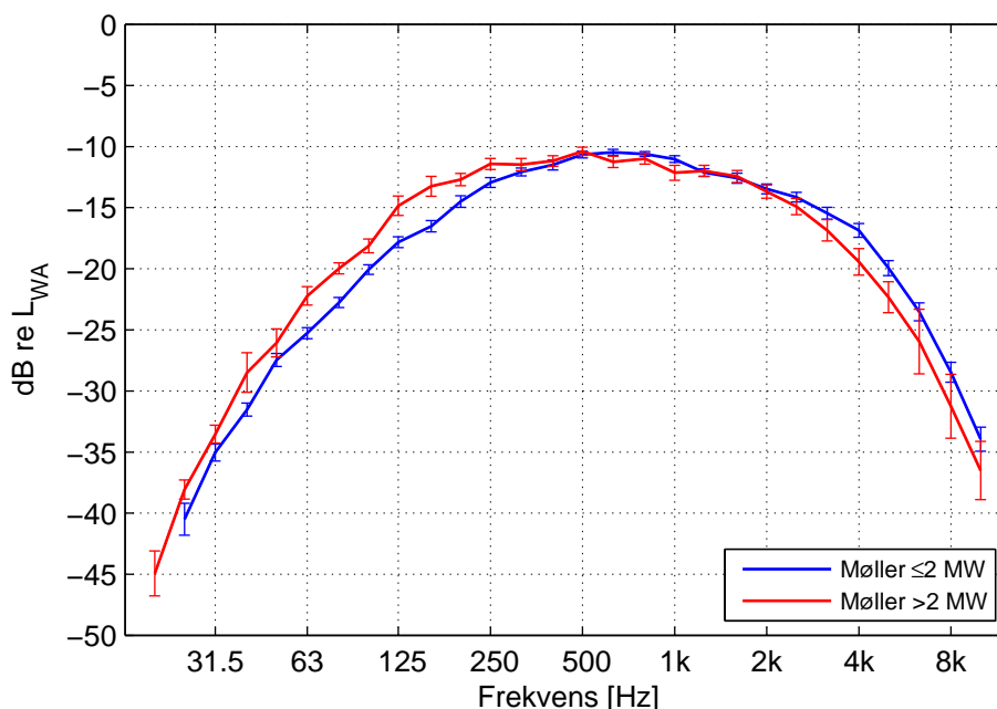
Figur 4. Normerede A-vægtede lydeffektniveauer i 1/3-oktavnå. Middelværdier for to grupper af møller: \leq 2 MW og > 2 MW. Lodrette streger angiver \pm 1 standard error of mean (s.e.m.).
