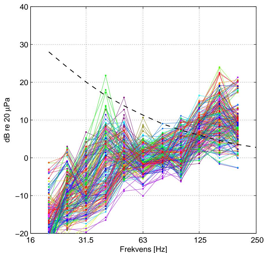
Figur 11. Indendørs A-vægtede lydtrykniveauer for 1/3-oktavnånd i den afstand fra hver enkelt mlle, hvor det totale A-vægtede lydtrykniveau udendrs er 35 dB (se Tabel 1). 207 kombinationer af 23 store mller og 9 rum. Den stiplede linje er hretrsklen i henhold til ISO 389-7 [29]. Farverne angiver mllen, farvekode som i Figur 5.
