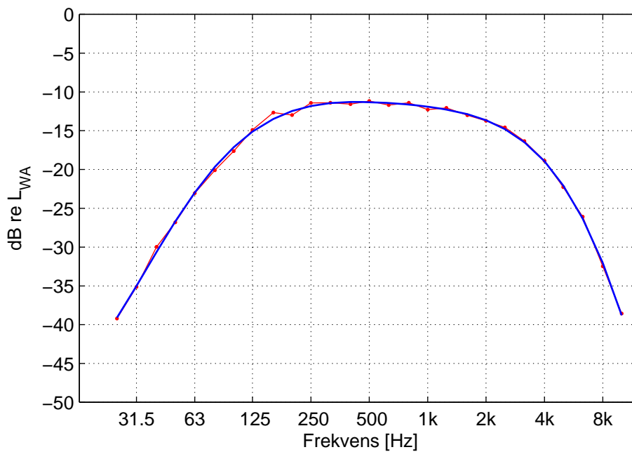
Figur 18. Sjette-ordens-polynomie regression (blå linje) af gennemsnit af normerede A-vægtede lydeffektniveauer (rød linje med runde markeringer) for møller med nominal elektrisk effekt > 2 MW.
